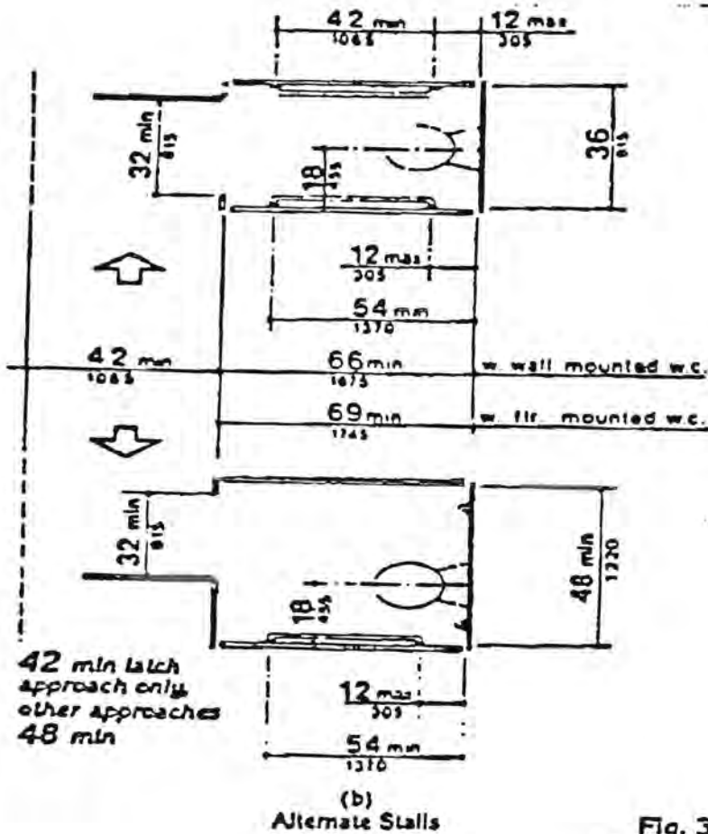
Fig. 30 Toilet Stalls
