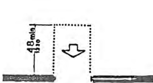
(d) Front Approach — Sliding Doors and Folding Doors
